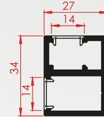
Profil Kodu:2037 Kg/m 0,695
