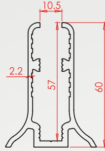
Profil Kodu: 1796 Kg/m 1,133
