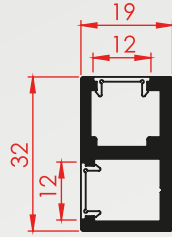
Profil Kodu:2036 Kg/m 0,554
