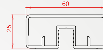
Profil Kodu:1869 Kg/m 0,941
