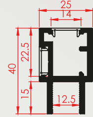
Profil Kodu:2032 Kg/m 0,738
