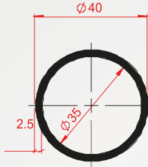
Profil Kodu:1260 Kg/m 0,799
