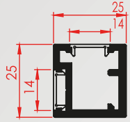
Profil Kodu:2033 Kg/m 0,545
