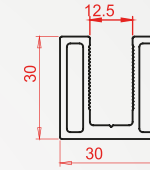
Profil Kodu: 2039 Kg/m 0,877
