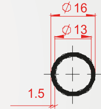
Profil Kodu:1074 Kg/m 0,184
