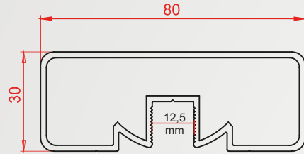
Profil Kodu:1870 Kg/m 1,200
