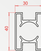
Profil Kodu:1872 Kg/m 0,805
