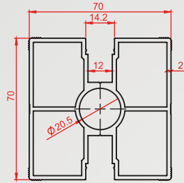
Profil Kodu:2040 Kg/m 2,551
