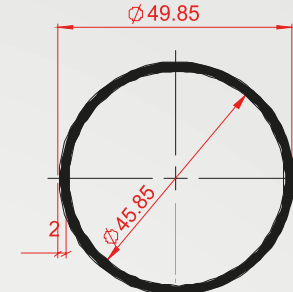
Profil Kodu:1784 Kg/m 0,816
