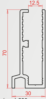
Profil Kodu: 1874 Kg/m 1,290
