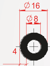
Profil Kodu:1075 Kg/m 0,409
