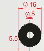
Profil Kodu:1282 Kg/m 0,491
