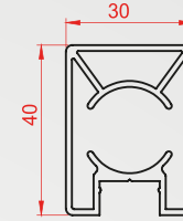
Profil Kodu:1873 Kg/m 0,829
