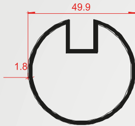
Profil Kodu:1041 Kg/m 0,870
