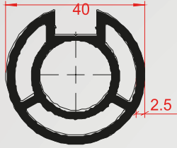
Profil Kodu:2099 Kg/m 1,329
