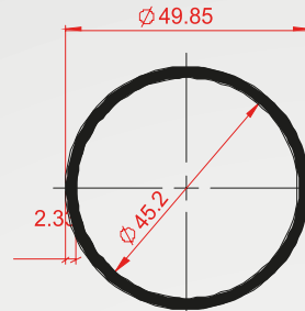
Profil Kodu:1004 Kg/m 0,940
