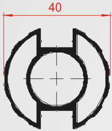
Profil Kodu:1006 Kg/m 0,797
