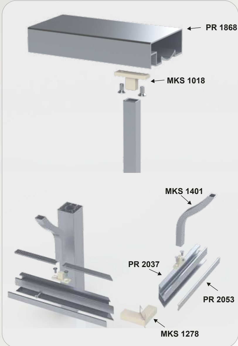
MODEL MKS 022 -KESİT
