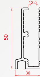
Profil Kodu: 2093 Kg/m 0,949
