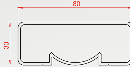
Profil Kodu:2094 Kg/m 1,073
