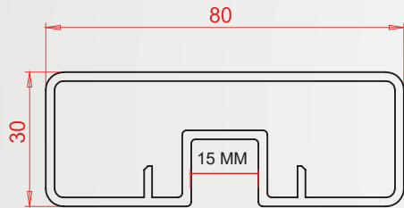
Profil Kodu:2168 Kg/m 1,348
