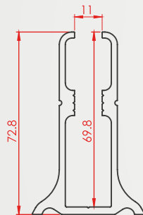
Profil Kodu:1042 Kg/m 1,716
