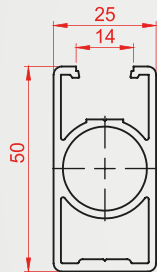
Profil Kodu: 2159 Kg/m 0,988
