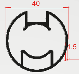
Profil Kodu:1005 Kg/m 0,770
