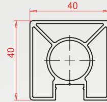
Profil Kodu:1817 Kg/m 1,060
