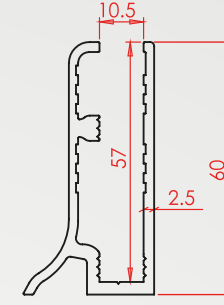
Profil Kodu: 1989 Kg/m 1,046
