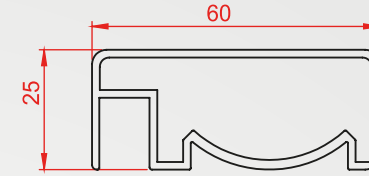
Profil Kodu:1198 Kg/m 0,867
