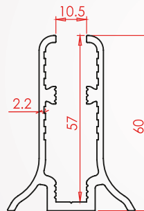
Profil Kodu:1796 Kg/m 1,133
