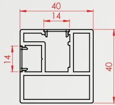
Profil Kodu:2098 Kg/m 1,144
