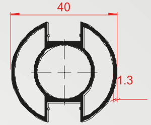
Profil Kodu:1602 Kg/m 0,748
