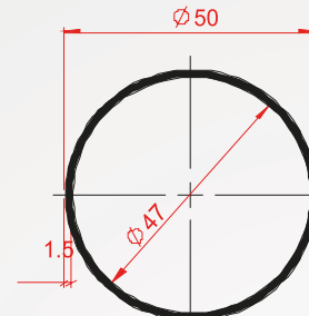
Profil Kodu:1261 Kg/m 0,621
