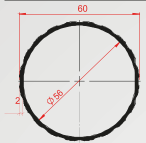
Profil Kodu:1040 Kg/m 0,900
