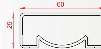
Profil Kodu:1867 Kg/m 0,845
