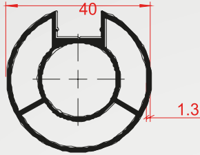
Profil Kodu:1044 Kg/m 0,759
