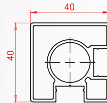
Profil Kodu:1818 Kg/m 0,965
