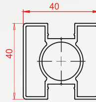
Profil Kodu:1816 Kg/m 0,965
